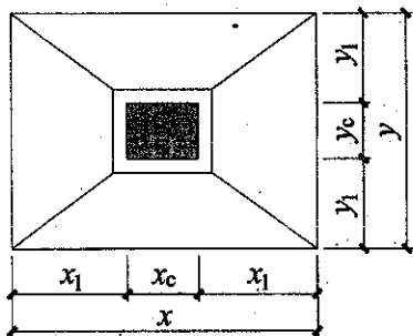
图 2.3.3-4 对称坡形截面普通独立基础原位标注
