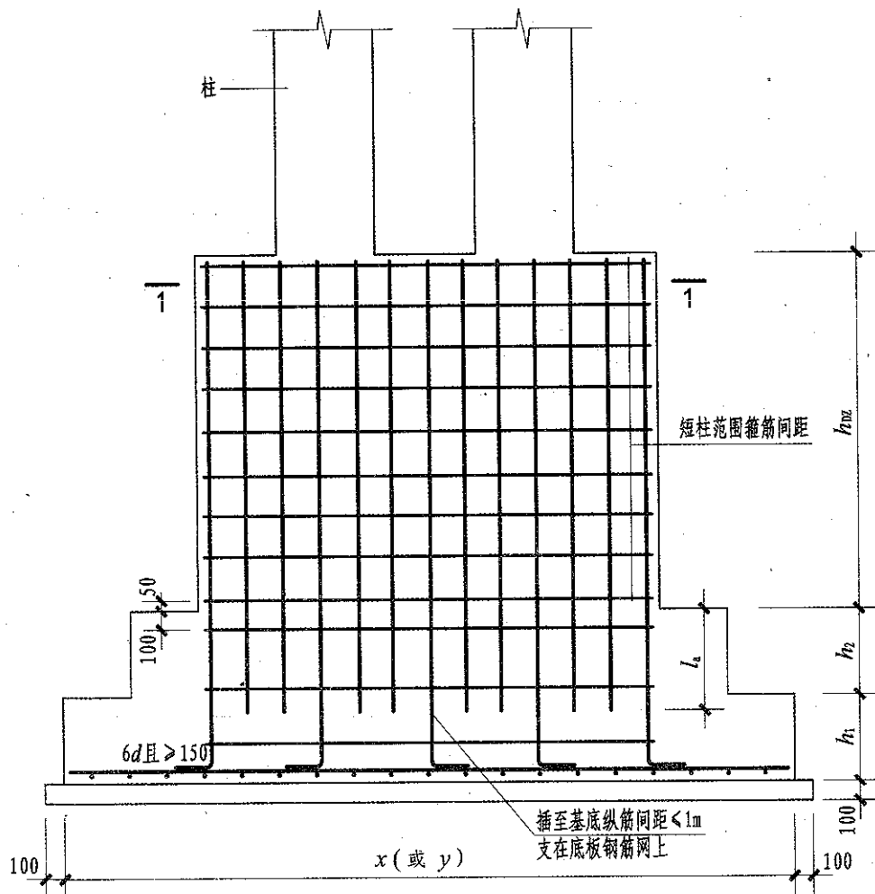
双柱普通独立深基础短柱配筋构造
