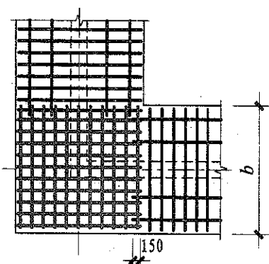
(转角梁板端部无纵向延伸)
