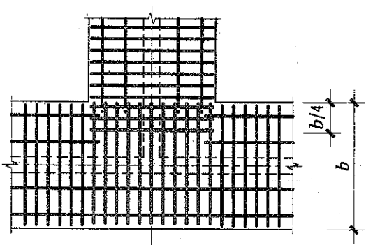
(丁字交接基础底板)
