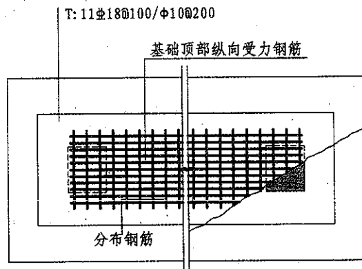
图 2.3.6-1 双柱独立基础顶部配筋示意
