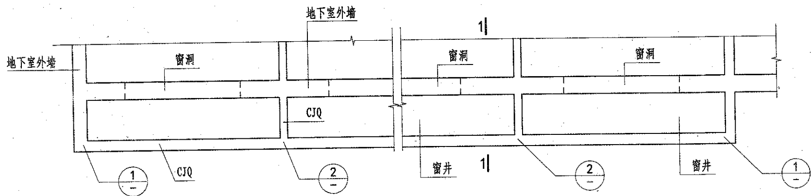
窗井平面布置图
