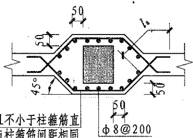
基础梁中心穿柱侧腋构造
