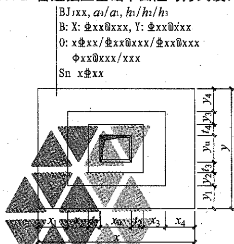
图 2.3.5 杯口独立基础平面注写方式设计表达示意
