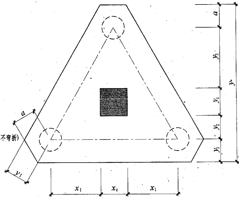
等边三桩承台CT J 配筋构造
