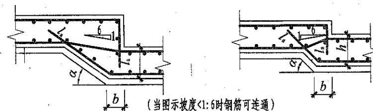
基坑JK构造
