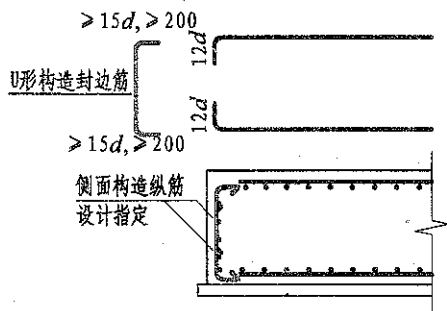
(a) U形筋构造封边方式
