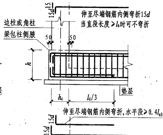
端部无外伸构造
