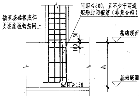
柱插筋在基础中锚固构造(一)
