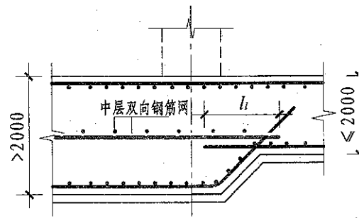
(c) 板底不一平
