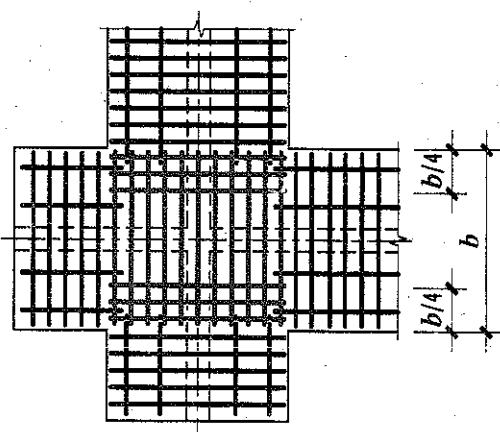
(转角梁板端部均有纵向延伸)
