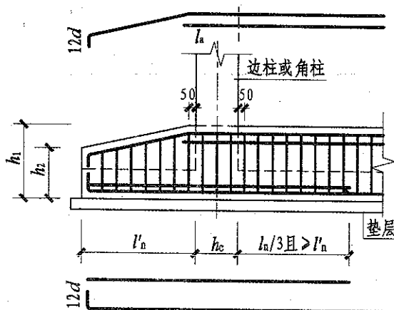
端部变截面外伸构造
