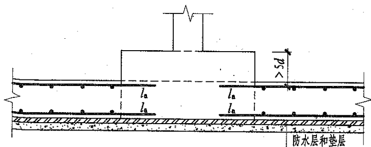
低板位防水底板(二)
