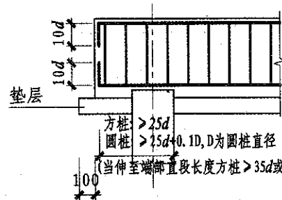
承台梁端部钢筋构造
