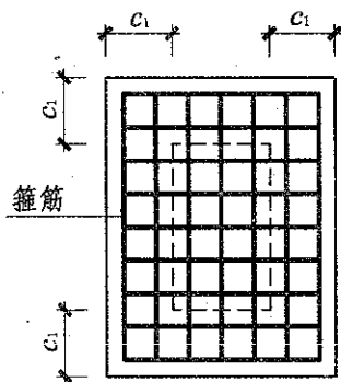
(矩形截面)
