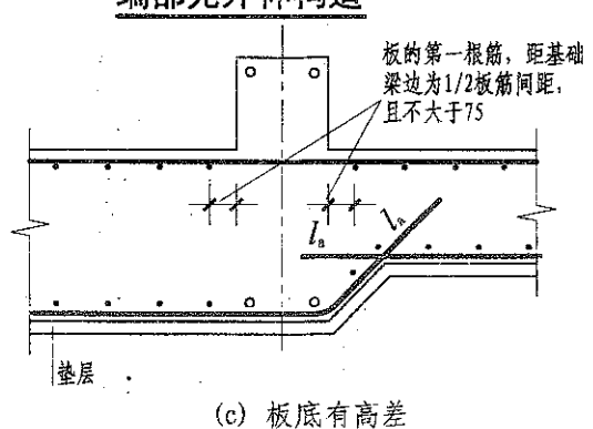
端部无外伸构造
