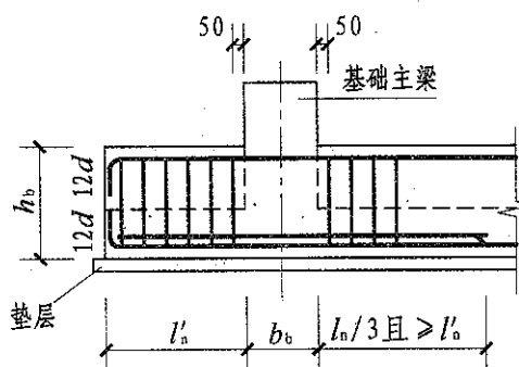
端部等截面外伸构造
