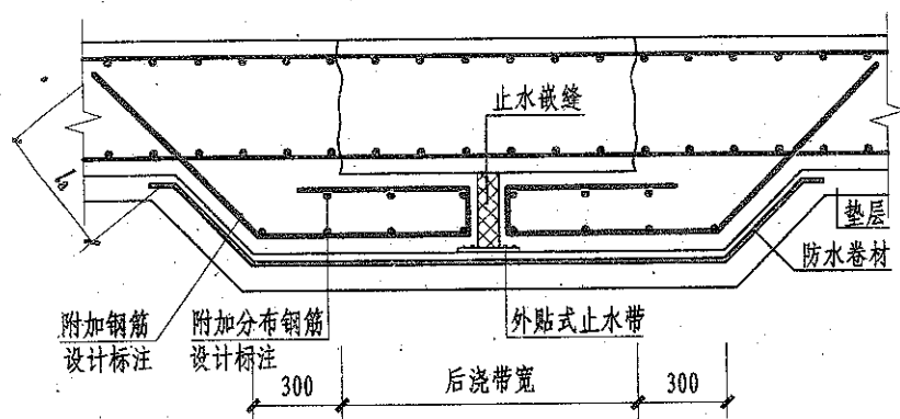
后浇带HJD超前止水构造
