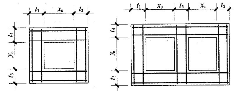
杯口顶部焊接钢筋网
