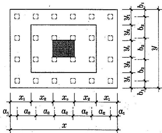
图 6.3.3-1 矩形独立承台平面原位标注
