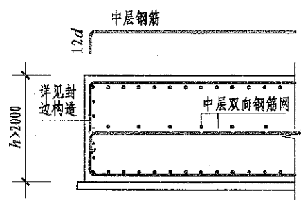
中层筋端头构造
