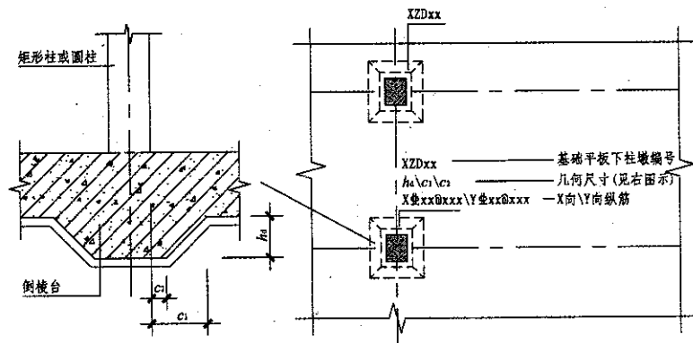
图 7.2.4-1 棱台形下柱墩引注图示
