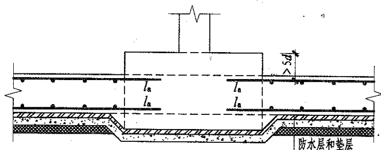
中板位防水底板(二)
