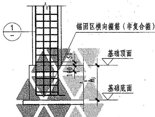
柱插筋在基础中锚固构造(四)
