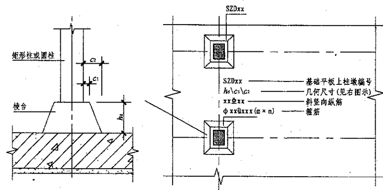
图 7.2.3-1 棱台形上柱墩引注图示
