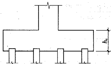
图 6.3.2-2 单阶截面独立承台竖向尺寸
