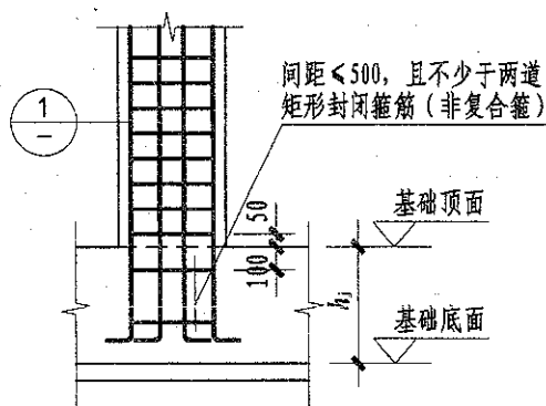
柱插筋在基础中锚固构造(二)
