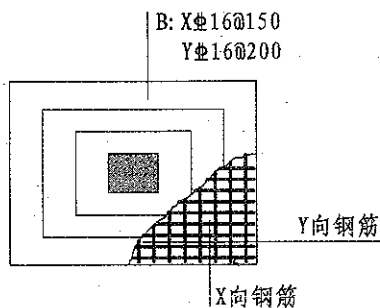
图 2.3.2-10 独立基础底板底部双向配筋示意
