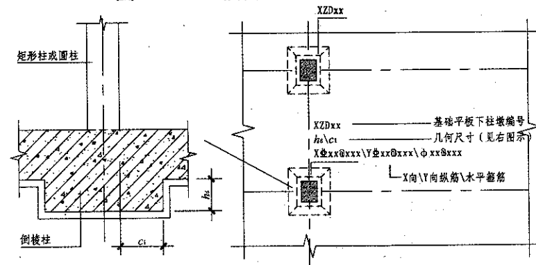
图 7.2.4-2 棱柱形下柱墩引注图示
