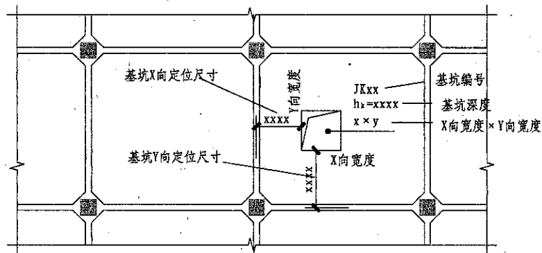
图 7.2.5 基坑 JK 引注图示
