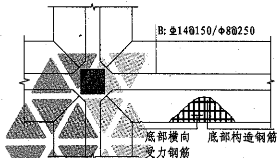
图 3.5.2-3 条形基础底板底部配筋示意
