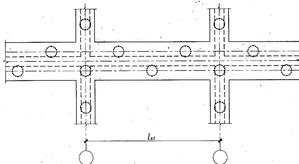
承台梁端部钢筋构造
