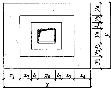
图 2.3.3-6 阶形截面杯口独立基础原位标注（一）
