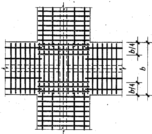
(十字交接基础底板)
