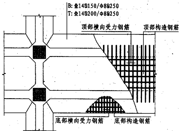
图 3.5.2-4 双梁条形基础底板顶部配筋示意
