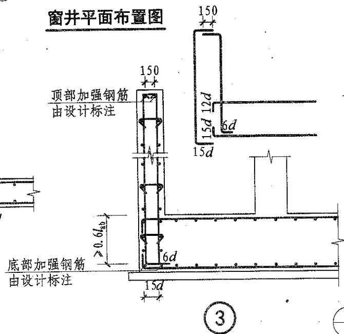
窗井墙CJQ配筋构造
