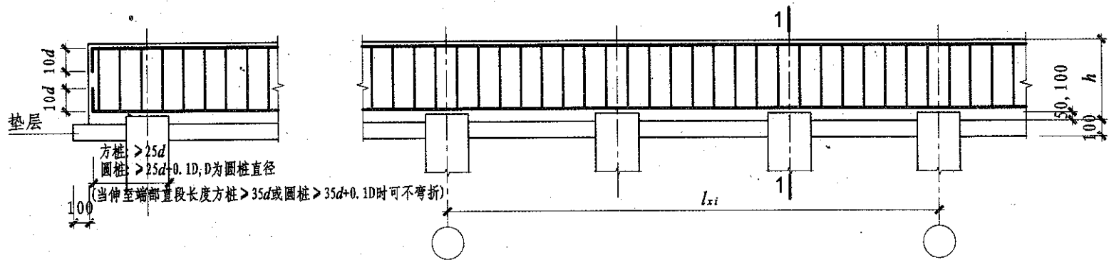
承台梁端部钢筋构造
