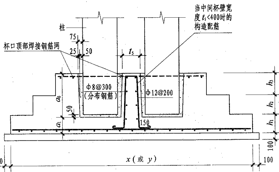
双杯口独立基础构造
