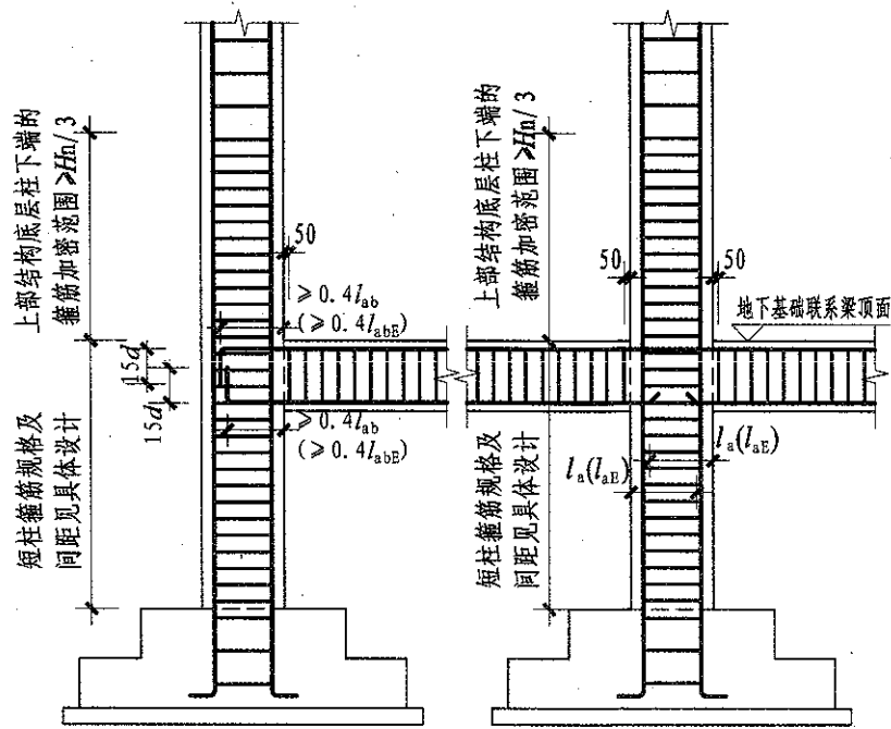
基础联系梁JLL配筋构造 (二)
