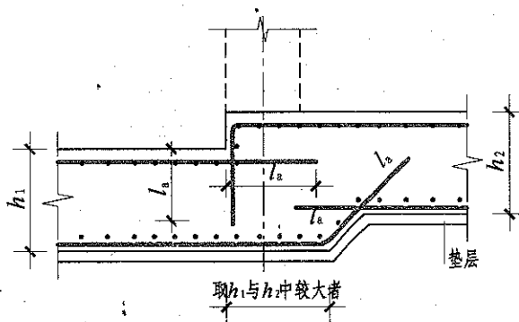
(b) 板顶、板底均有高差
