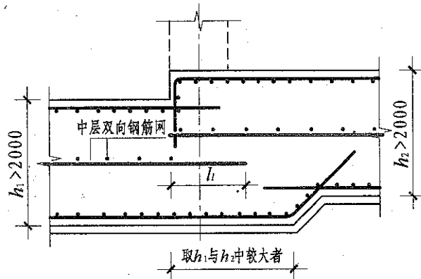
(b) 板顶、板底均不一平
