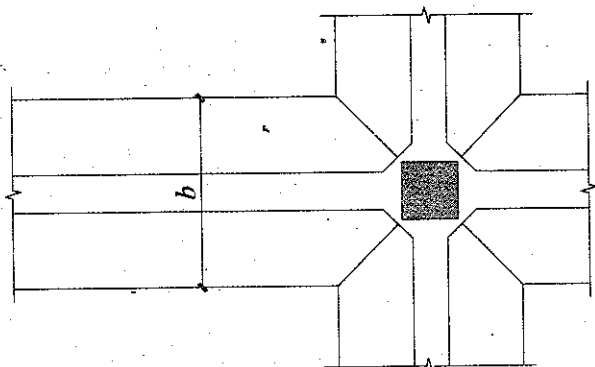
图 3.5.3 条形基础底板平面尺寸原位标注 梁板式条形基础存在双梁共用同一基础底板、墙下条形
