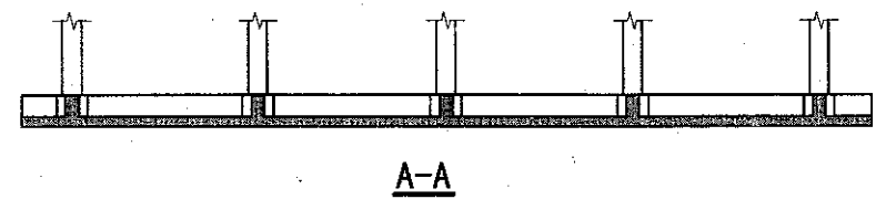
梁板式筏形基础平板LPB标注图示
