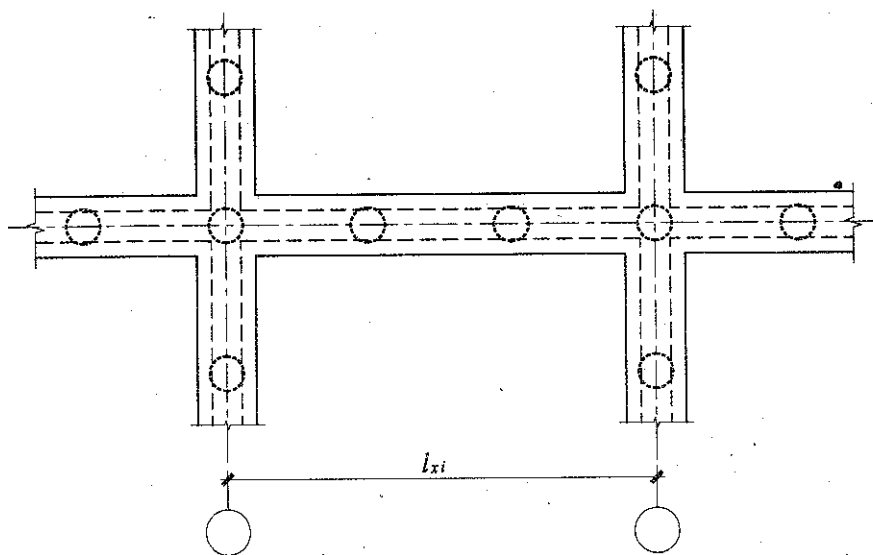
承台梁端部钢筋构造
