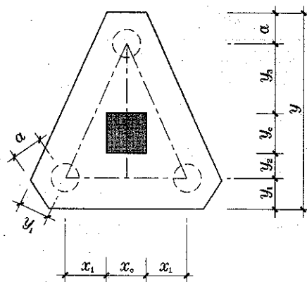
图 6.3.3-3 等腰三桩独立承台平面原位标注
