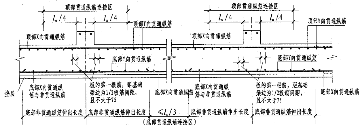
梁板式筏形基础平板LPB钢筋构造
