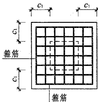
(正方形截面)
