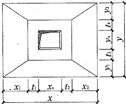
图 2.3.3-8 坡形截面杯口独立基础原位标注 (一)
