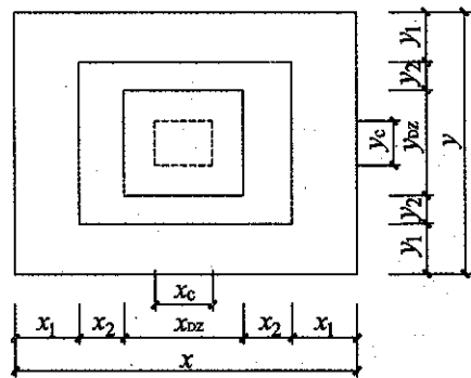
图 2.3.3-3 设置短柱独立基础的原位标注
