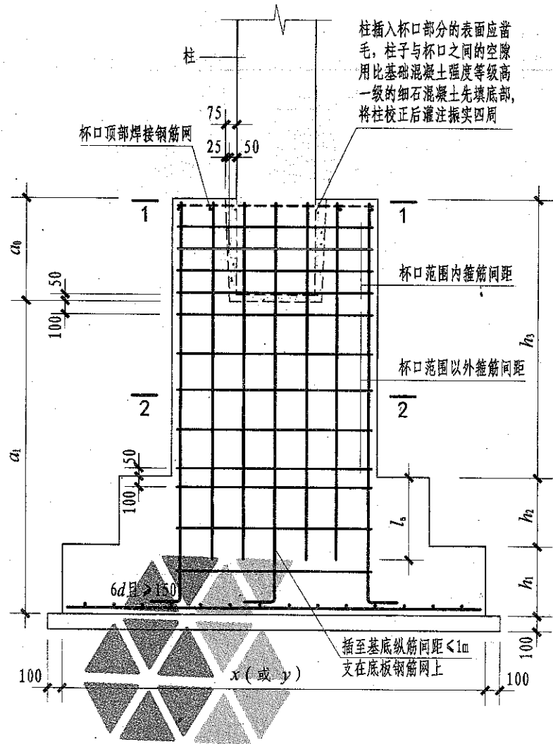
高杯口独立基础杯壁和基础短柱配筋构造
