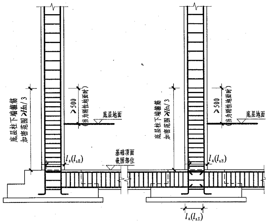
基础联系梁JLL配筋构造 (一)
