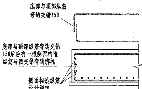
(b) 纵筋弯钩交错封边方式
