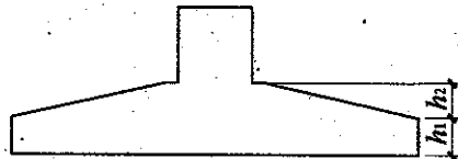
图 3.5.2-1 条形基础底板坡形截面竖向尺寸
