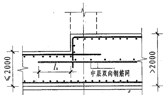
(a) 板顶不一平
