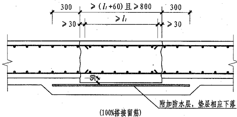
基础底板后浇带HJD构造
