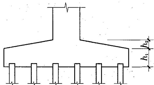
图 6.3.2-3 坡形截面独立承台竖向尺寸
