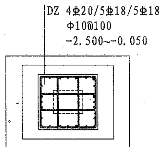
图 2.3.2-15 独立基础短柱配筋示意
