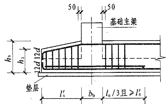
端部变截面外伸构造
