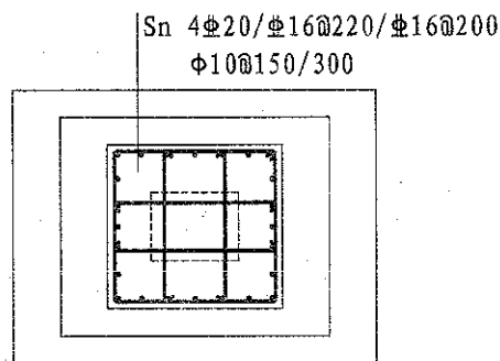
图 2.3.2-13 高杯口独立基础杯壁配筋示意
