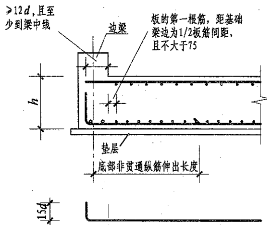
端部无外伸构造 (二)
