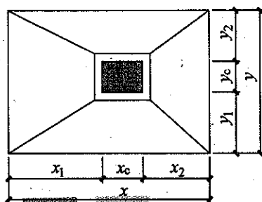
图 2.3.3-5 非对称坡形截面普通独立基础原位标注
