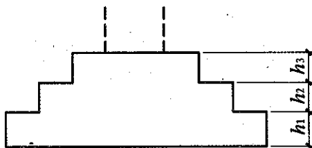
图 2.3.2-1 阶形截面普通独立基础竖向尺寸
