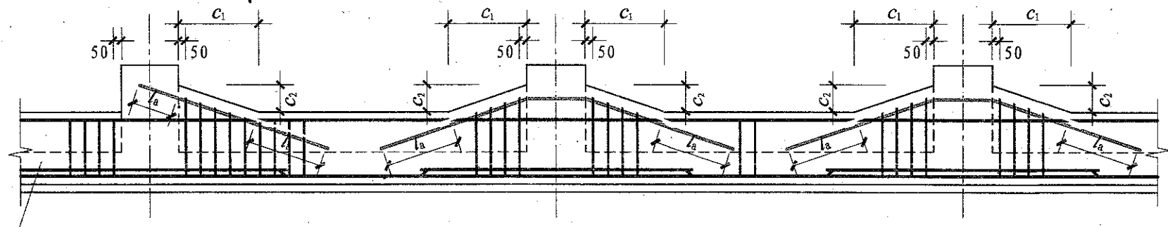
基础次梁JCL竖向加腋钢筋构造
