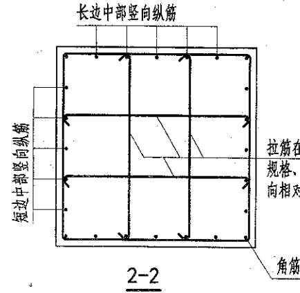
高杯口独立基础杯壁和基础短柱配筋构造
