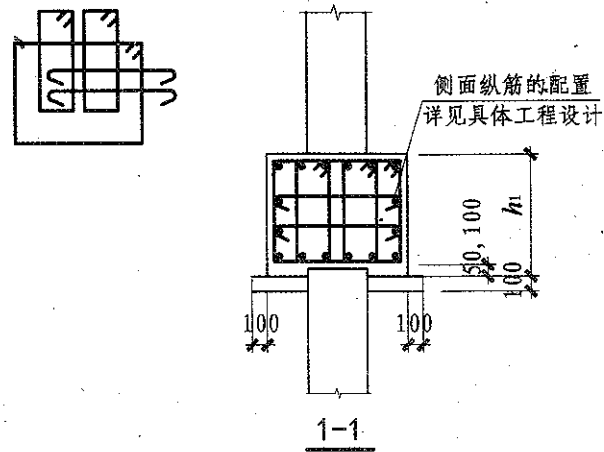
墙下单排桩承台梁CTL配筋构造
