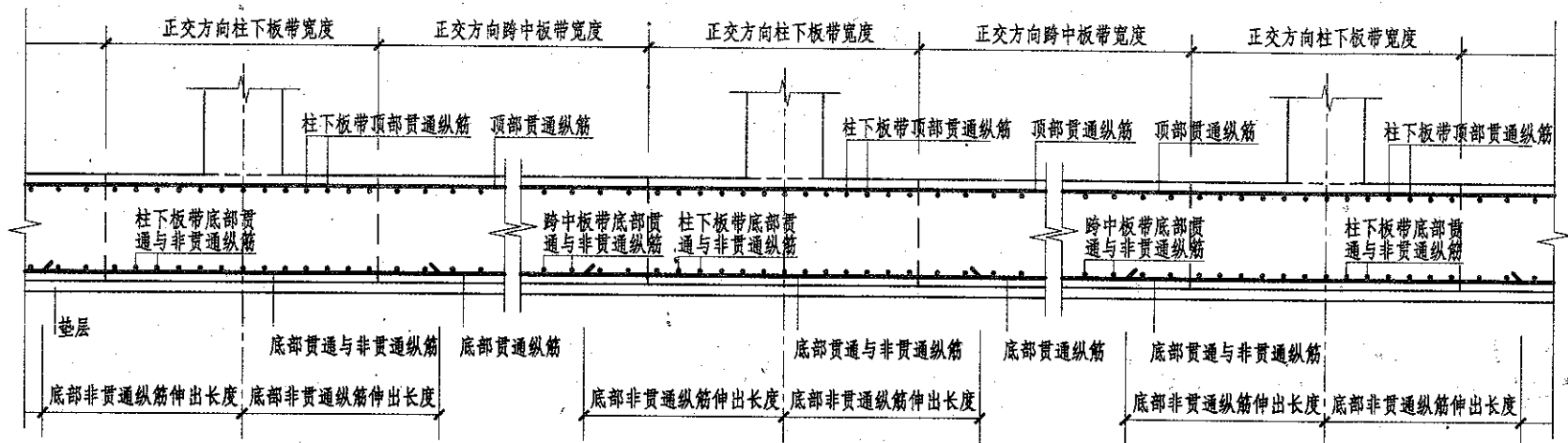
平板式筏基柱下板带ZXB纵向钢筋构造
