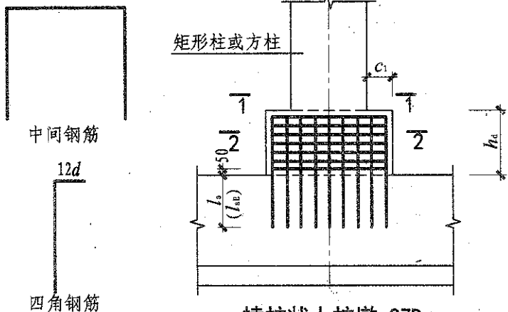
棱柱状上柱墩 SZD
