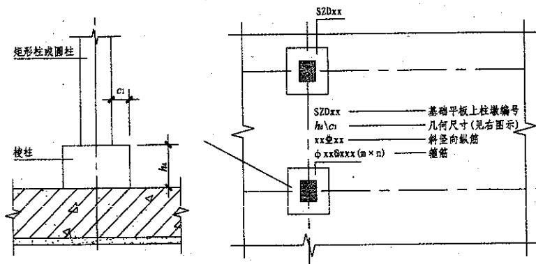
图 7.2.3-2 棱柱形上柱墩引注图示
