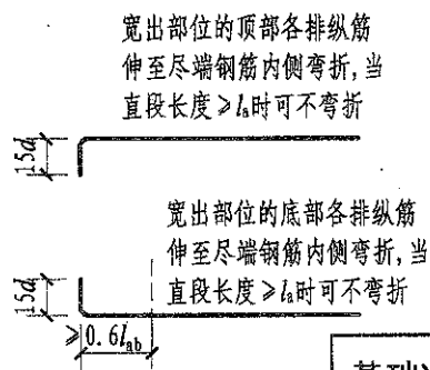
支座两边梁宽不同钢筋构造
