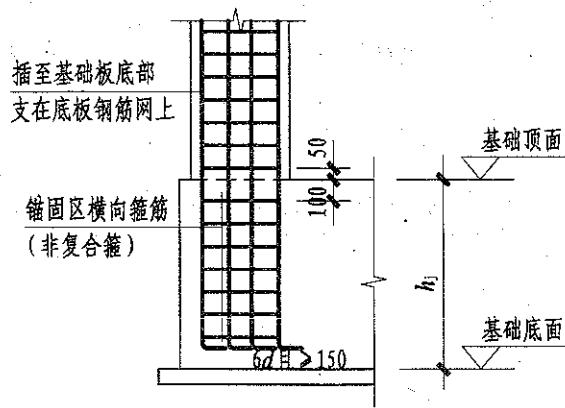
柱插筋在基础中锚固构造(三)
