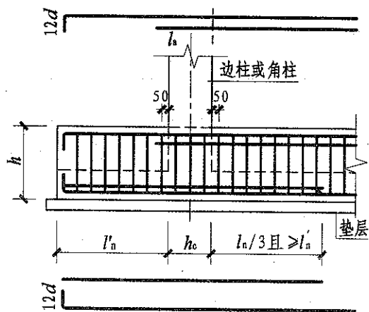
端部等截面外伸构造
