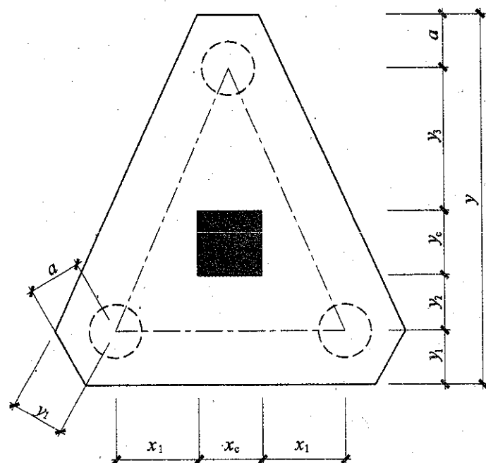
等腰三桩承台CTJ配筋构造
