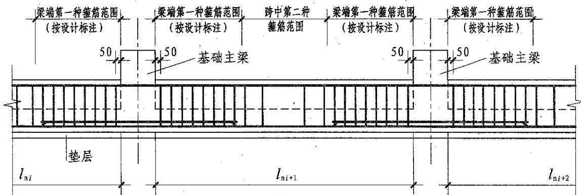
基础次梁JCL配置两种箍筋构造
