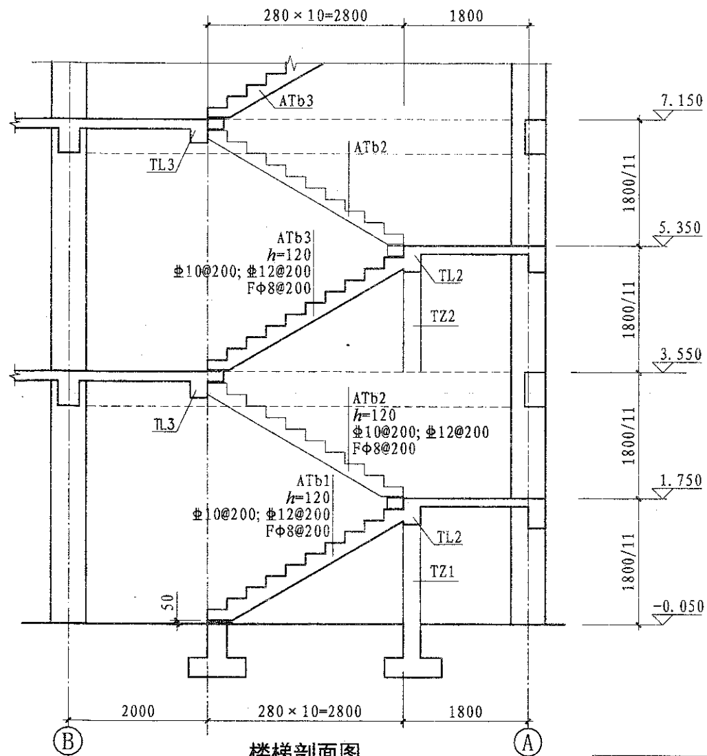
楼梯剖面图
