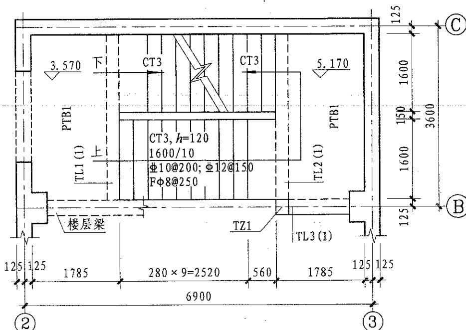
图2 设计示例 \nabla 3.570— \nabla 5.170楼梯平面图
