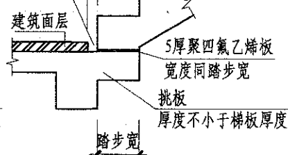
(2) 设聚四氟乙烯垫板 (梯段浇筑时应在垫板上铺塑料薄膜)
