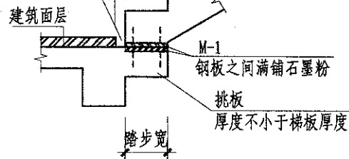
(1) 预埋钢板
