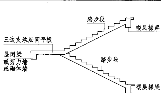
HT型（有层间平台板的双跑楼梯）
