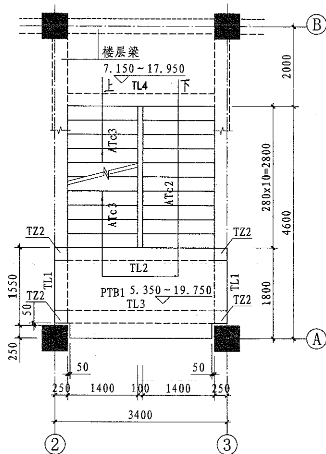
标准层平面图
