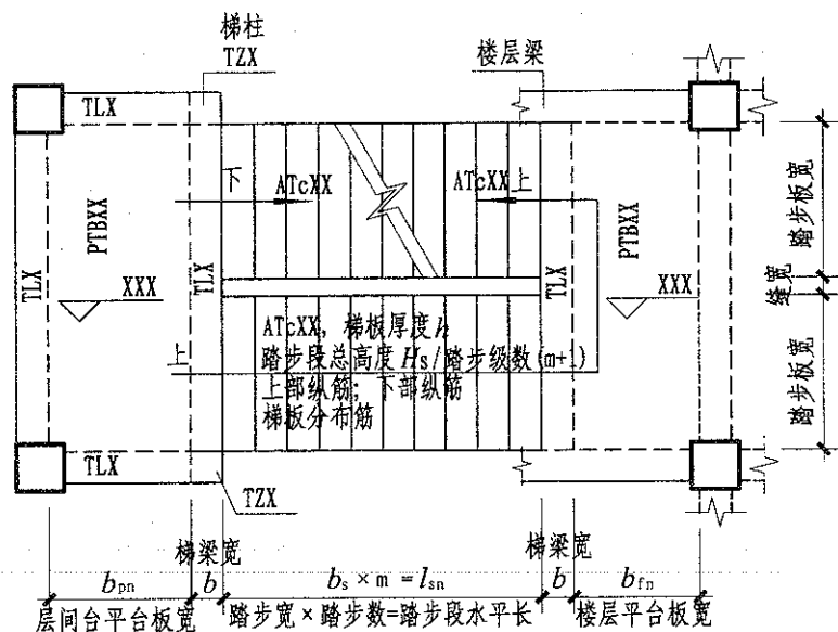
图1 注写方式 标高XXX—标高XXX楼梯平面图 (楼梯休息平台与主体结构整体连接)
