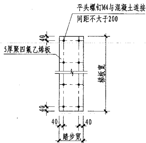
聚乙烯四氟板
