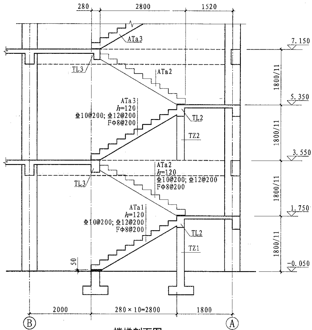
楼梯剖面图
