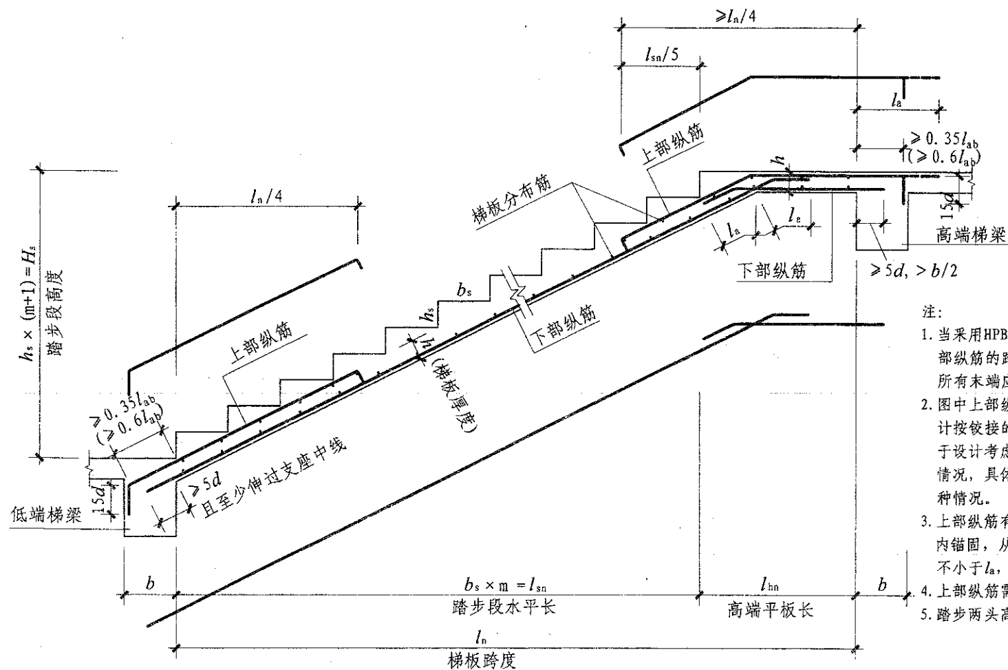
CT型楼梯板配筋构造
