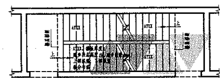
图4 交叉楼梯(无层间平台板)
