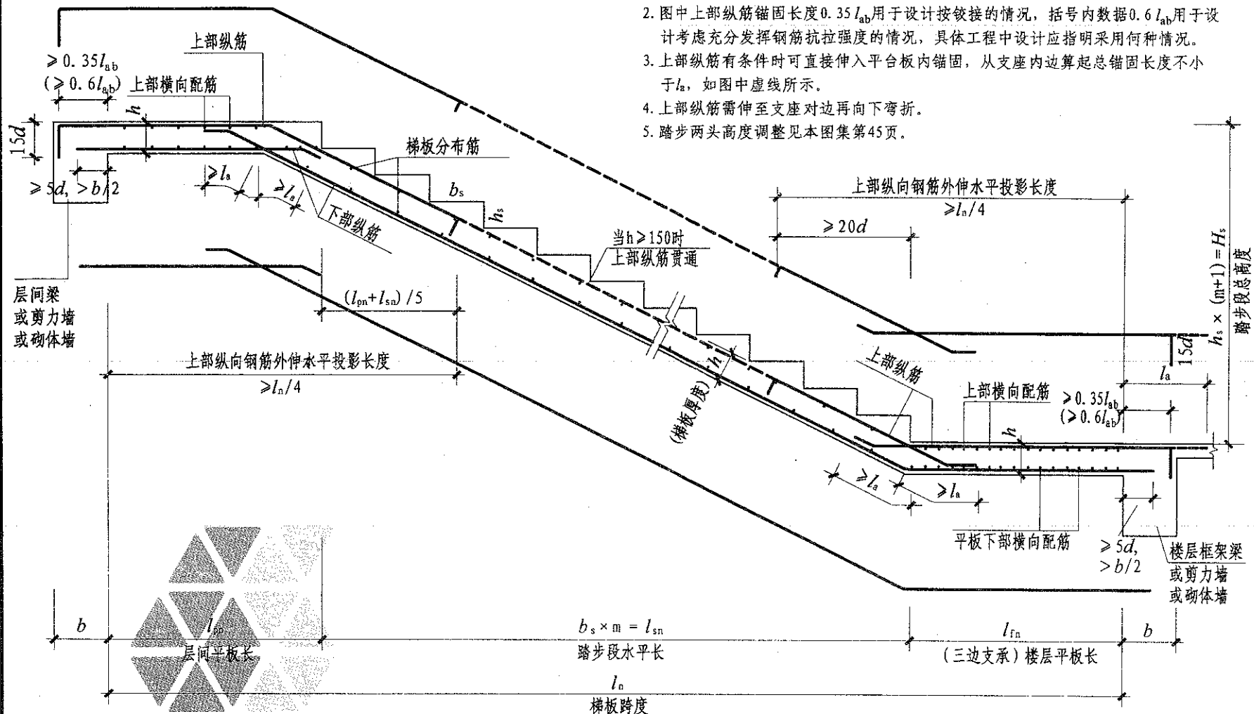
GT楼梯板配筋构造 (A-A)
