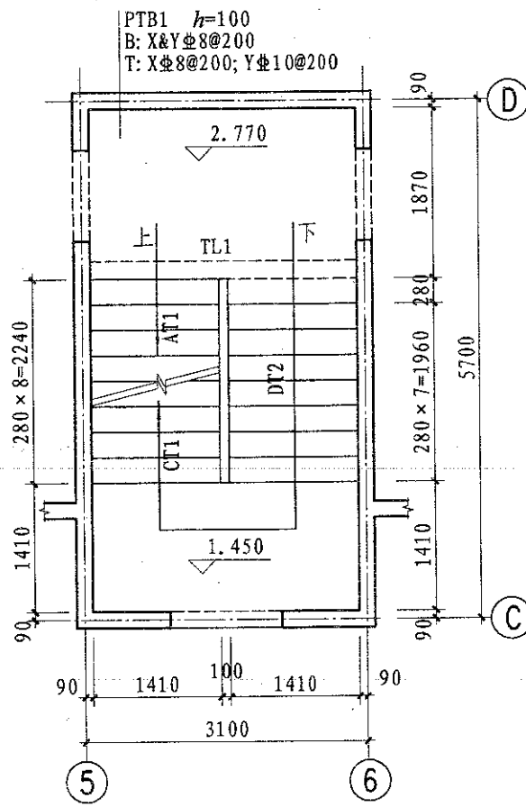
▽ 1.450 ~ 2.770 楼梯平面图
