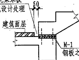
(1) 预埋钢板
