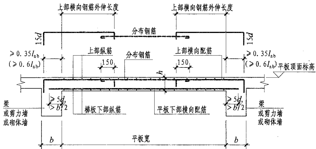
C-C剖面楼梯平板配筋构造
