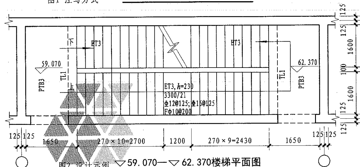
标高XXX—标高XXX楼梯平面图
