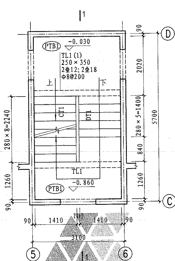
▽ -0.860 ~ -0.030 楼梯平面图
