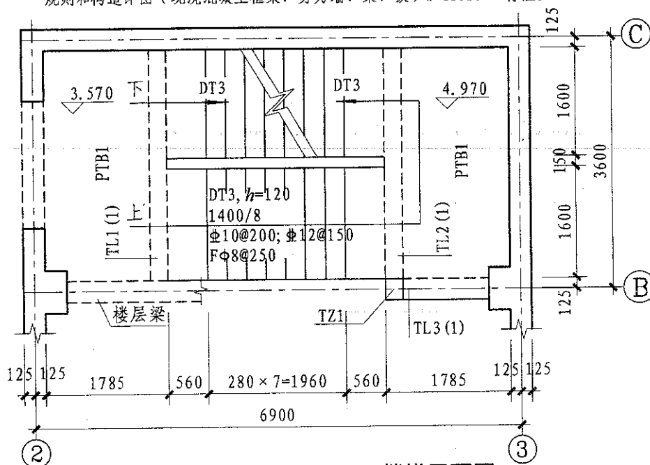
图2 设计示例 \nabla 3.570— \nabla 4.970楼梯平面图
