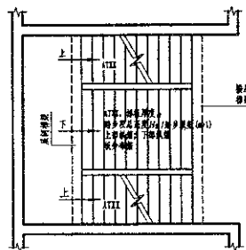
图3 双分平行楼梯
