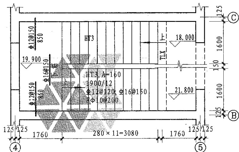
图2 设计示例 ▽18.000—▽21.800楼梯平面图
