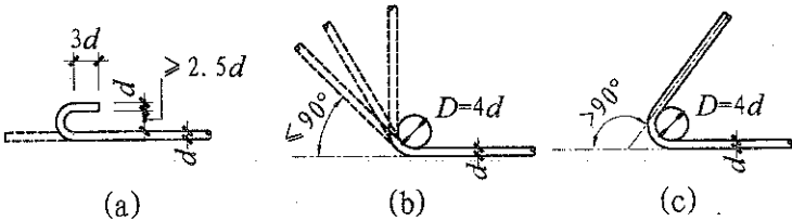
钢筋弯钩构造
