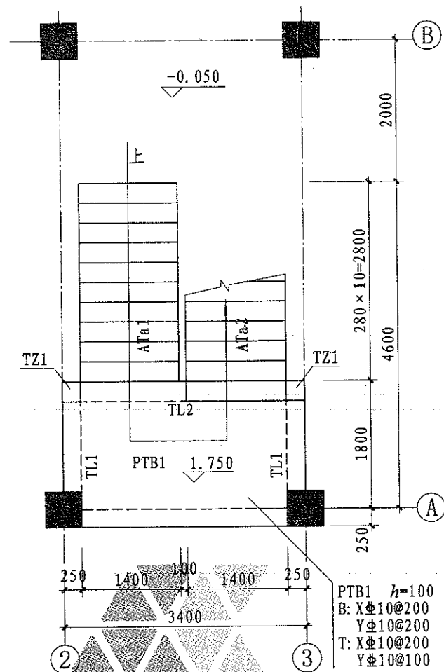
一层平面图
