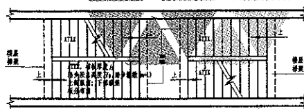
图5 剪刀楼梯
