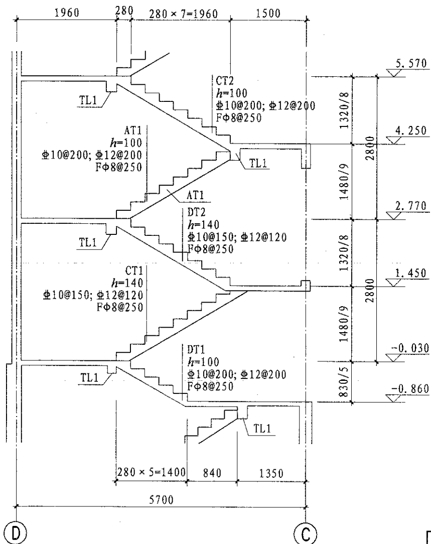
1-1剖面图
