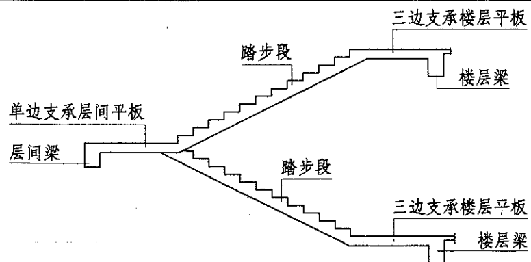
GT型（有层间和楼层平台板的双跑楼梯）
