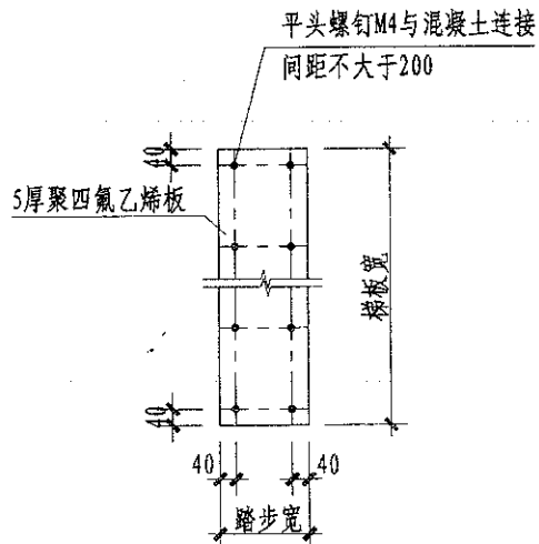
聚四氟乙烯板
