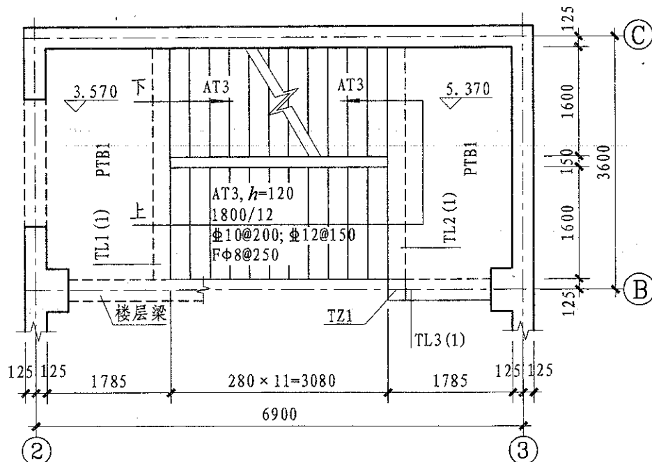
图2. 设计示例 \nabla 3.570— \nabla 5.370楼梯平面图
