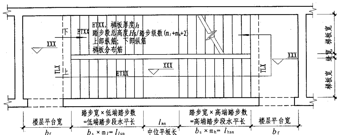
标高XXX—标高XXX楼梯平面图
