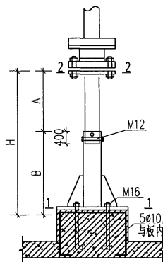
ZGU-III型针在屋面上安装
