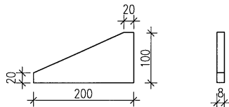
2号零件
