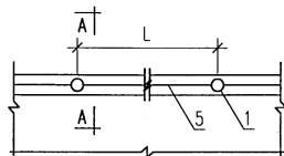
女儿墙防雷平面(局部)
