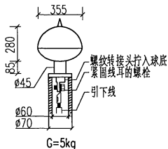
S3000针外形尺寸图
