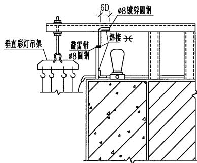
垂直彩灯顶部防雷做法
