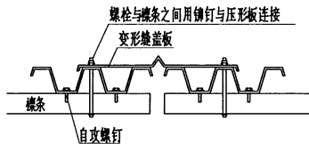
伸缩缝处安装图
