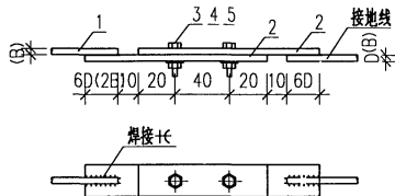
断接卡 (一)
