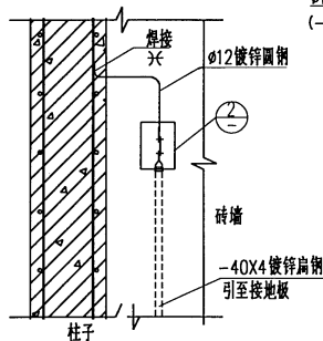
暗装断接卡子做法(二)
