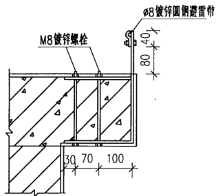
① 节点
