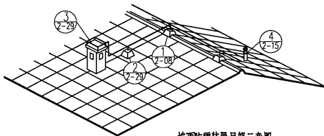
坡顶防雷装置局部示意图
