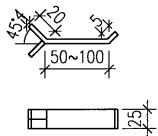
固定钩
