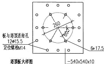
塔顶板大样图
