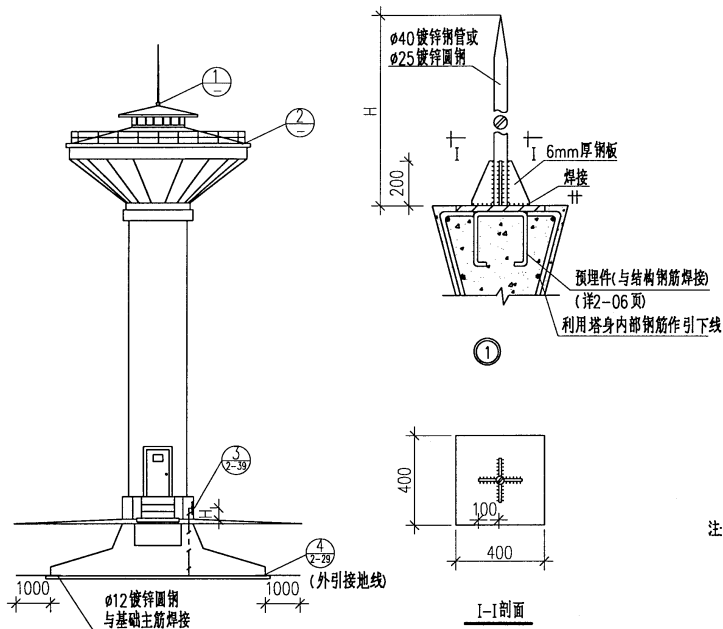
水塔避雷做法
