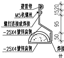
②脊瓦上的防雷做法(二)
