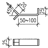
(10a)固定钩
