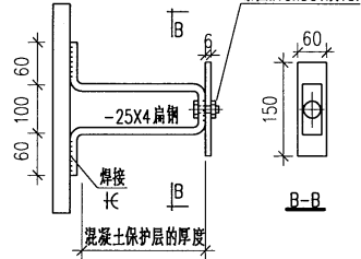
预埋连接板做法B
