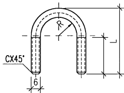
管卡 3
