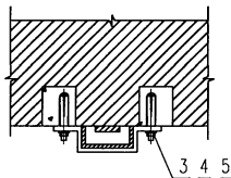
引下线保护(II)
