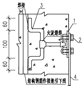
接地端子板安装做法(一)
