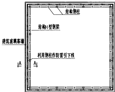
楼层平面图
