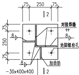
塔脚板连接大样
