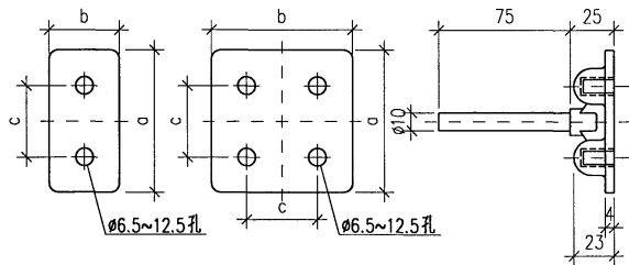
接地端子板外形图
