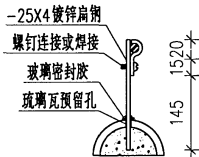
②脊瓦上的防雷做法(一)
