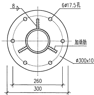
A01针在针塔上安装图
