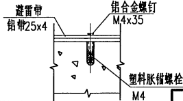
塑料胀锚螺栓 M4
