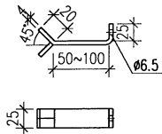
(10b)固定钩
