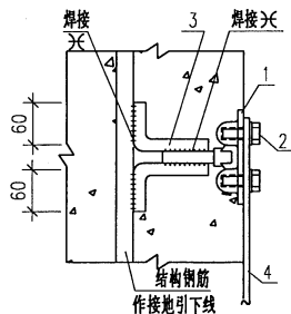
接地端子板安装做法(二)
