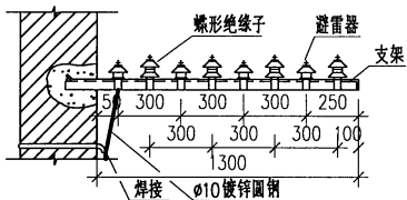
I型四线式(侧视)
