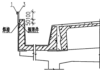
天沟上明装(一)
