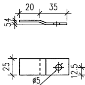
(3)S形卡子
