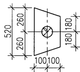
3号零件
