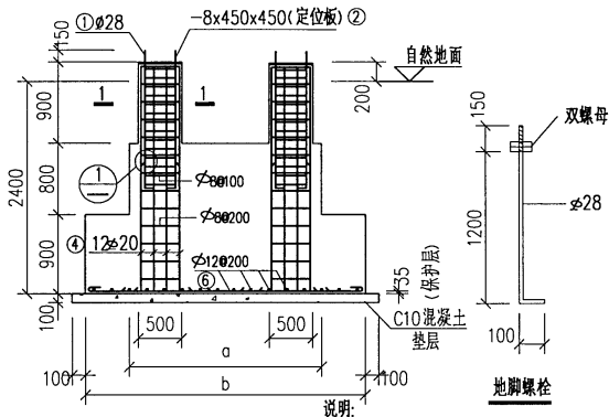
配筋图
