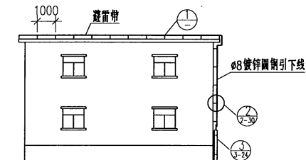
加气板平屋顶避雷带立面
