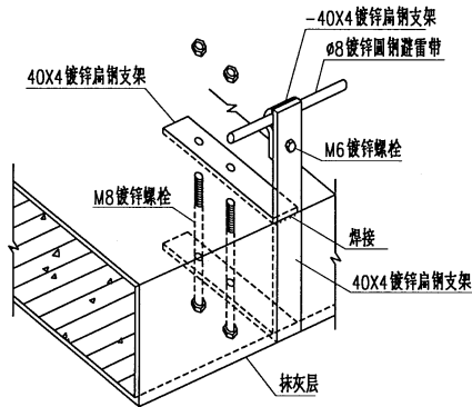
支架透视图
