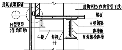
A-A剖面图
