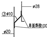
地脚螺栓与基础 钢筋焊接大样
