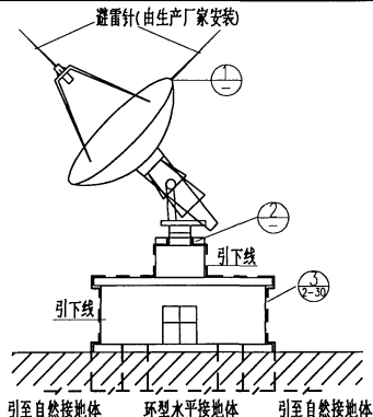
卫星地面站防雷接地示意图
