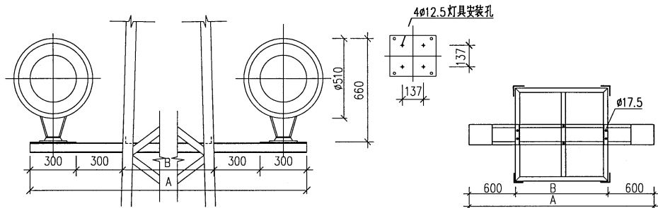
DLTG3型投光灯安装示意
