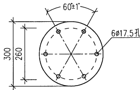
顶部法兰盘
