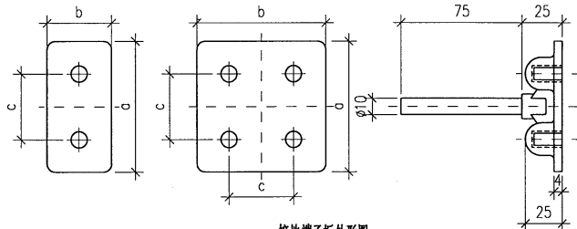
接地端子板外形图
