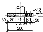
1-1 剖面
