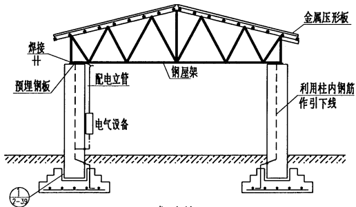
钢屋架剖面
