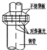
节点处外包不锈钢板大样图
