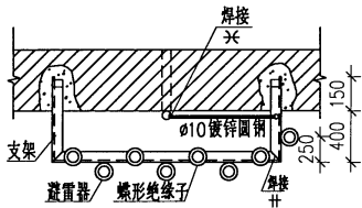
II型四线式(俯视)
