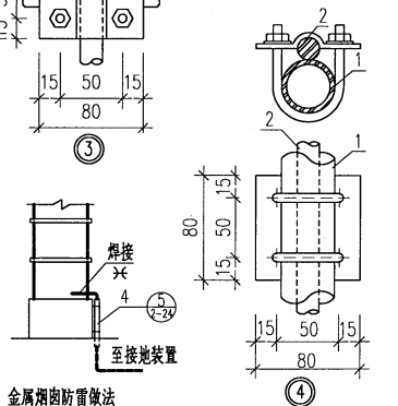
金属烟囱防雷做法
