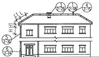
四坡顶防雷装置立面图
