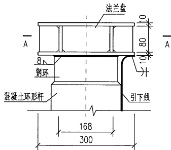
钢筋混凝土环形杆顶钢环 与法兰盘连接大样图
