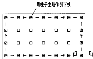
无防水层底板避雷接地极平面图
