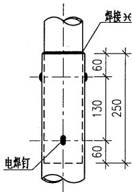
节点 IV
