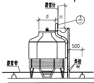
屋顶冷却塔防雷做法
