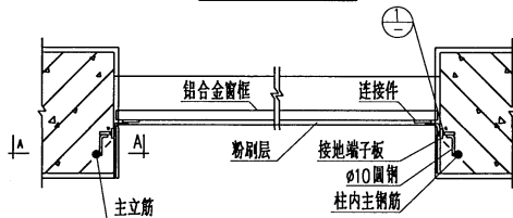
通长铝合金窗平面图
