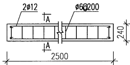
梁钢筋图
