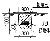
ZGD -II-1 型水平设置示意图
