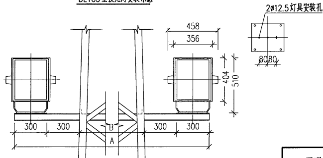
DLTG4型投光灯安装示意
