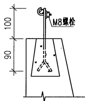
预制窗口支座做法
