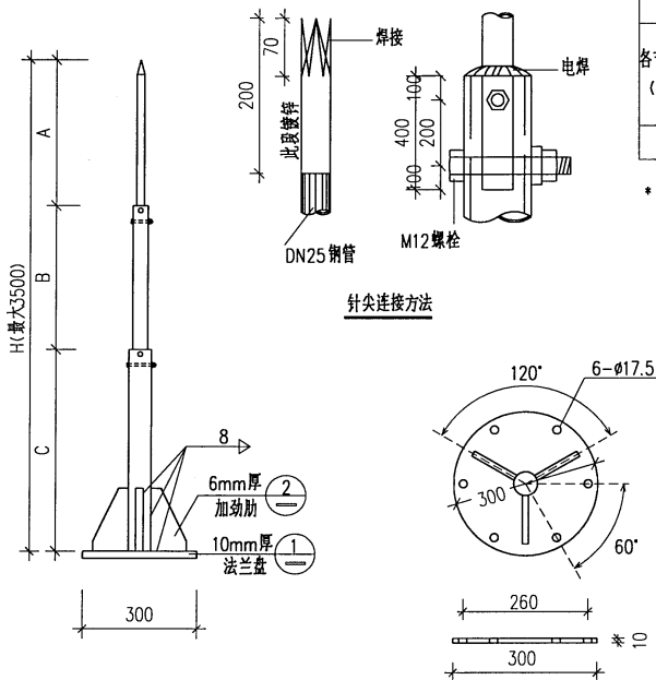
① 法兰盘
