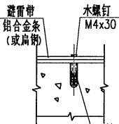
避雷带贴装
