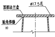
① 顶部法兰盘与钢管焊接大样
