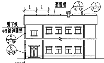
两坡顶防雷装置立面图
