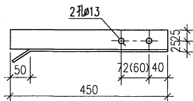
2号零件
