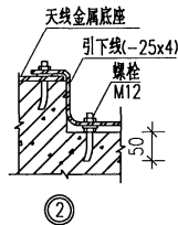
卫星地面站防雷接地示意图
