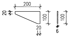
② 加肋
