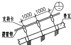
斜脊避雷帶做法
