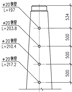
预埋钢管大样图
