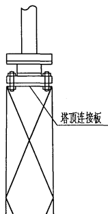
ZGU-III型针在角钢塔上安装
