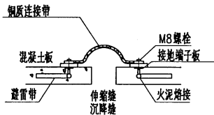
避雷带过伸缩缝做法 I
