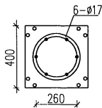
塔顶连接板 10mm 钢板
