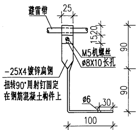
① 斜脊瓦支持卡做法
