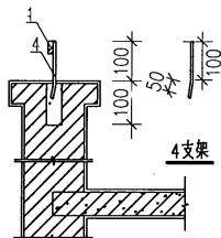
女儿墙上明装
