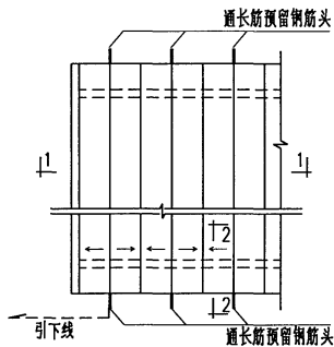
屋盖布置图(避雷带暗装)
