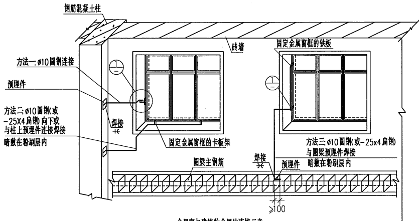
金属窗与建筑物金属体连接示意
