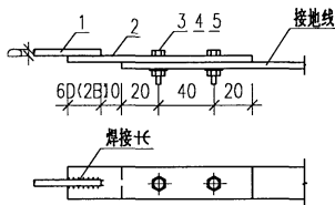
断接卡 (二)
