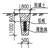
ZGD -I-3 型垂直设置示意图
