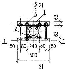
MT3-1 照明台构造图
