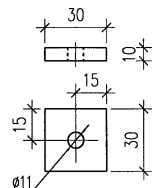
(7)垫片
