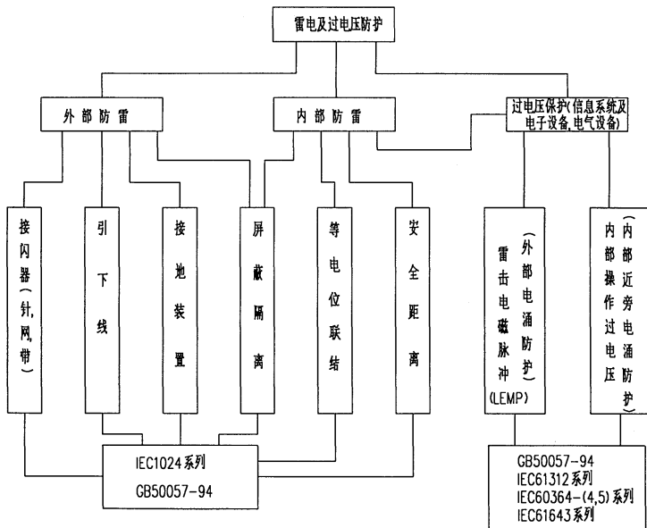
建筑物综合防雷系统方框图
