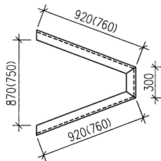
2号零件
