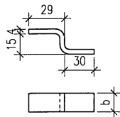
(9)S形卡子
