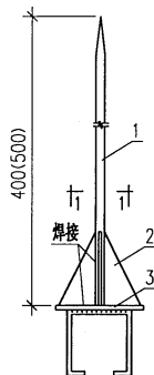
避雷短针立面
