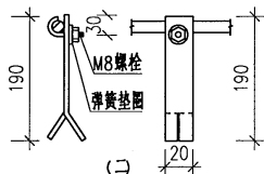
支持卡子
