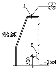
女儿墙上贴装
