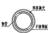
钢管外包不锈钢板大样图
