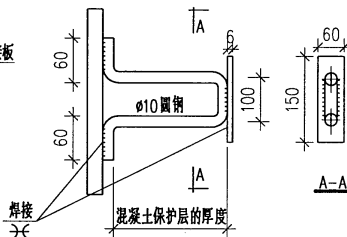
预埋连接板做法A
