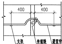
避雷带过伸缩缝做法 III
