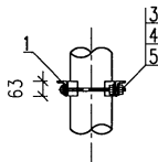
2-2 剖面
