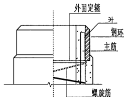
电杆顶部纵向钢筋 与钢环连接大样
