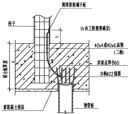
柱内扁钢与钢管桩锚筋焊接剖面图
