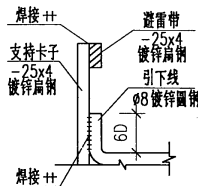
圆钢引下线连接
