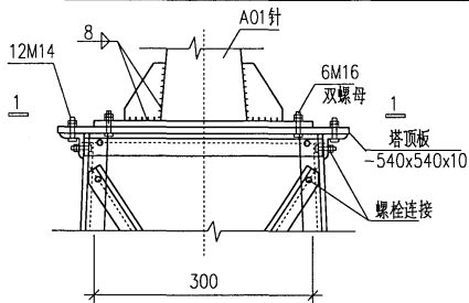
A01针在针塔上安装图
