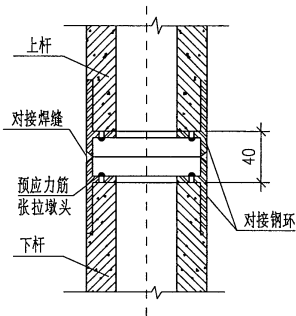
预应力环形混凝土杆
