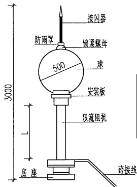
ZGU-III避雷针外形图
