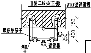
II型二线式(俯视)
