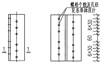
连结包铁大样图
