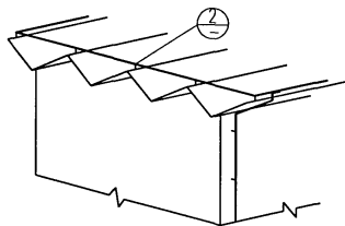
屋盖布置图(避雷带明装)
