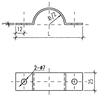
管卡 1
