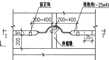
避雷带过伸缩缝做法 II
