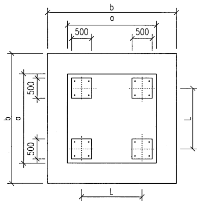
基础平面图
