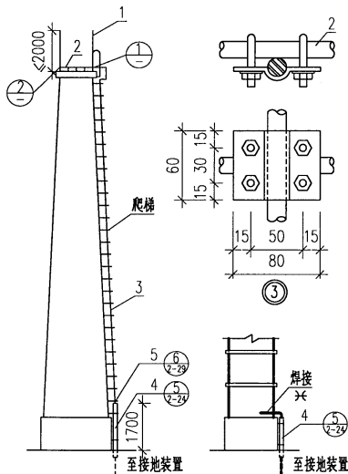
砖烟囱防雷做法
