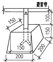
预制混凝土支座
