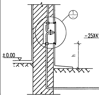
暗装断接卡子做法(一)
