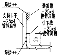
扁钢引下线连接
