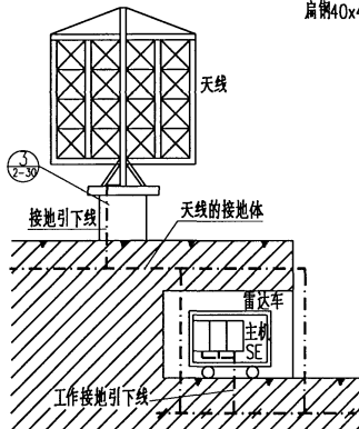
雷达站天线及机房防雷接地剖面图
