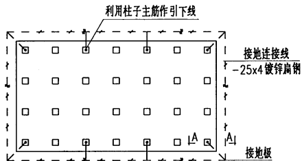
有防水层底板避雷接地极平面图
