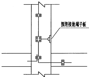
钢筋连接法示例
