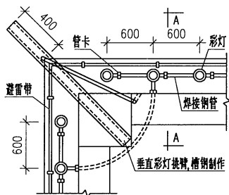
屋顶彩灯平面示意图
