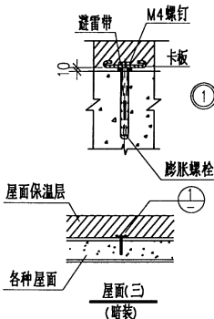
屋面(三) (暗装)
