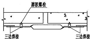
I-I剖面图
