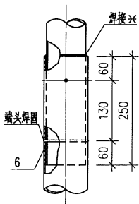
节点 I~III
