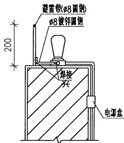
屋顶彩灯防雷做法
