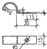
圆钢卡子
