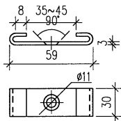
(6)卡板
