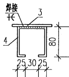
避雷短针做法
