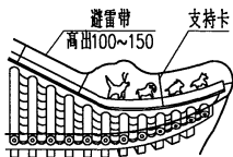
挑檐避雷带做法示意
