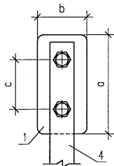
接地线安装做法
