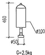
LCT针外形尺寸图
