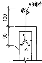
现浇窗口支座做法
