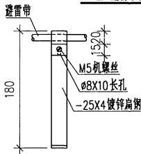
檐口避雷带做法
