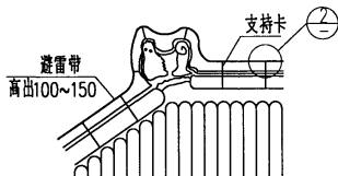
兽头及屋脊避雷带做法示意
