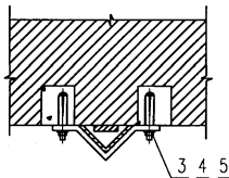
引下线保护(I)
