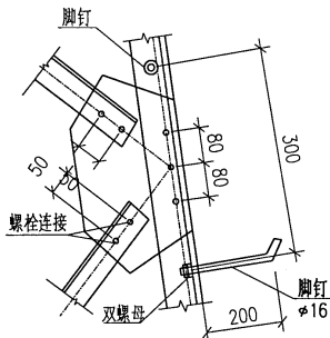
节点大样图
