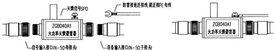
ZGB040A1 大功率天馈避雷器安装示意图
