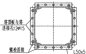
塔顶大样图
