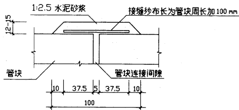
管块连接管带抹缝做法
