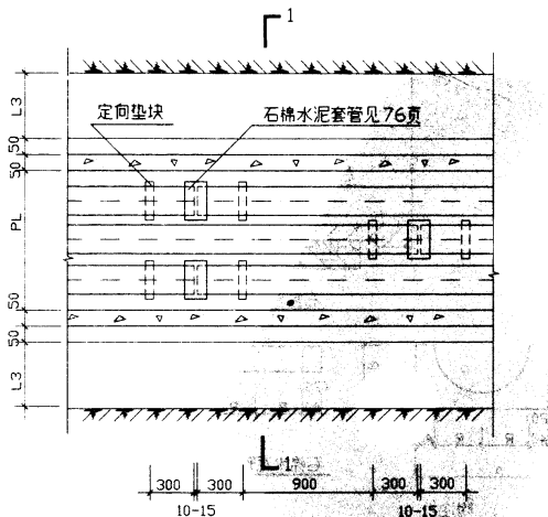
平面图
