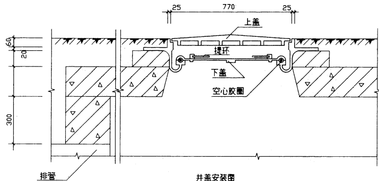
井盖安装图
