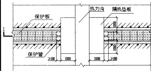
电缆与热力沟交叉(一)
