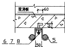
扁钢吊钩安装(二)
