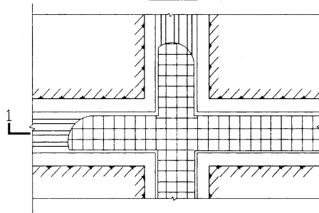
电缆与电缆交叉(一)
