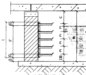
主架安装尺寸图
