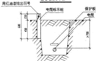
直埋电缆标示桩(-)
