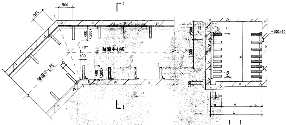
平面图
