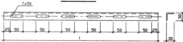
支 架 (三)
