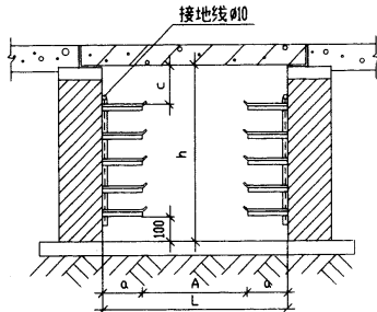
双侧支架电缆沟
