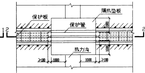
电缆与热力沟交叉敷设(二)
