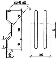
预埋件 2
