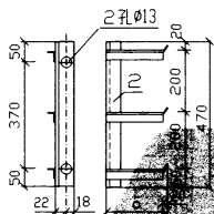
支架 2
