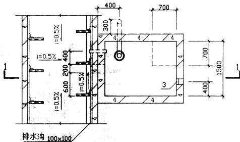
集水井平面
