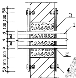
(一) 耐火隔板及矿棉封堵
