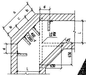
电缆沟转 90° (-)
