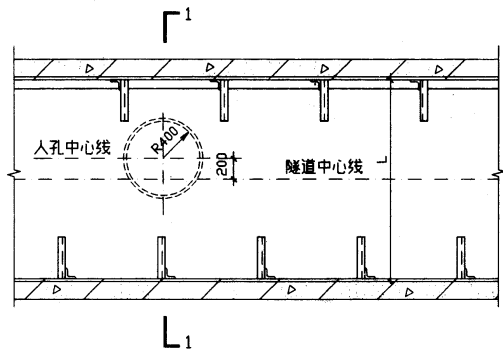
平面图
