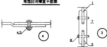
难燃封闭槽盒平面图
