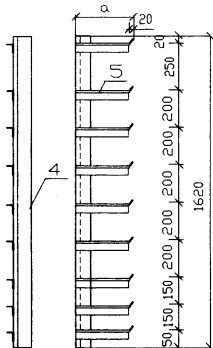
支架 1
