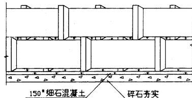
基础做法二 剖面图
