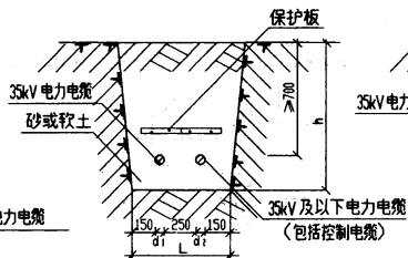
35kV 及以下电缆并列(一)
