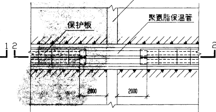
电缆与热力管道交叉(二)
