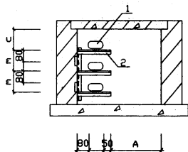
在电缆沟中安装
