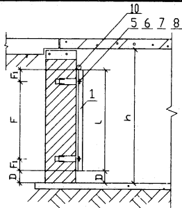
主架安装 (a)
