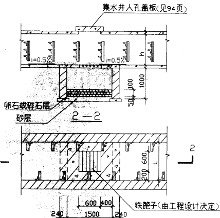
无覆盖层沟内集水井
