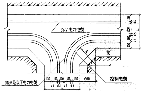
电缆直埋分支段(一)
