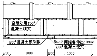
基础做法一 剖面图
