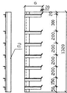
支架 2
