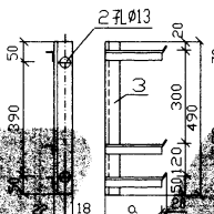
支架 3
