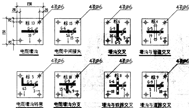
电缆壕沟标示牌
