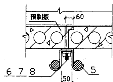
扁钢吊钩安装(三)
