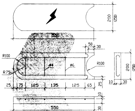
保护板(-)
