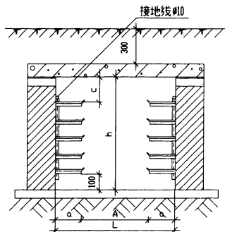
有覆盖层电缆沟
