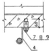
扁钢吊钩安装(二)
