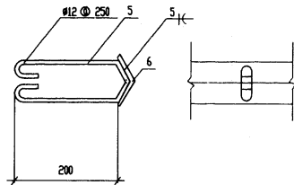
预埋件 3
