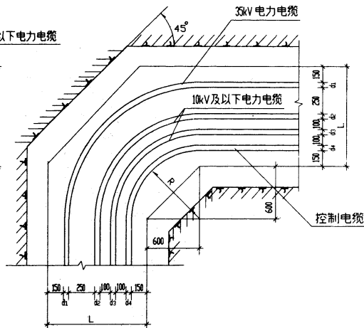
电缆直埋转 90°
