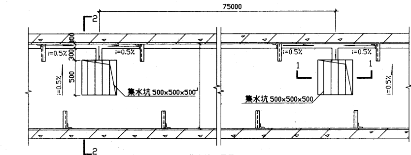
集水坑平面图
