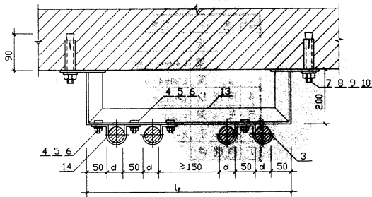
支架安装(二)
