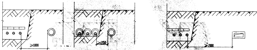
电缆与水管平行
