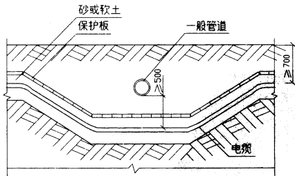
电缆与管道交叉(一)
