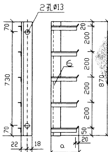
支架 6
