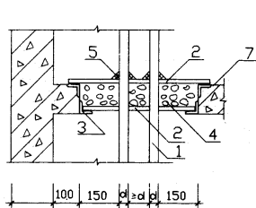
(一) 耐火隔板及矿棉封堵
