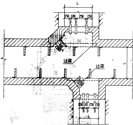
电缆沟分支段 (二)
