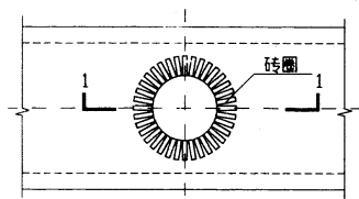
砖圈平面图
