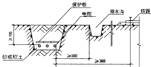
电缆与铁路平行
