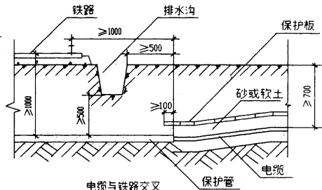
电缆与铁路交叉
