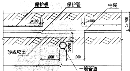
电缆穿管与管道交叉(二)
