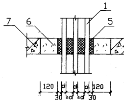
(二) 速固型堵料封堵
