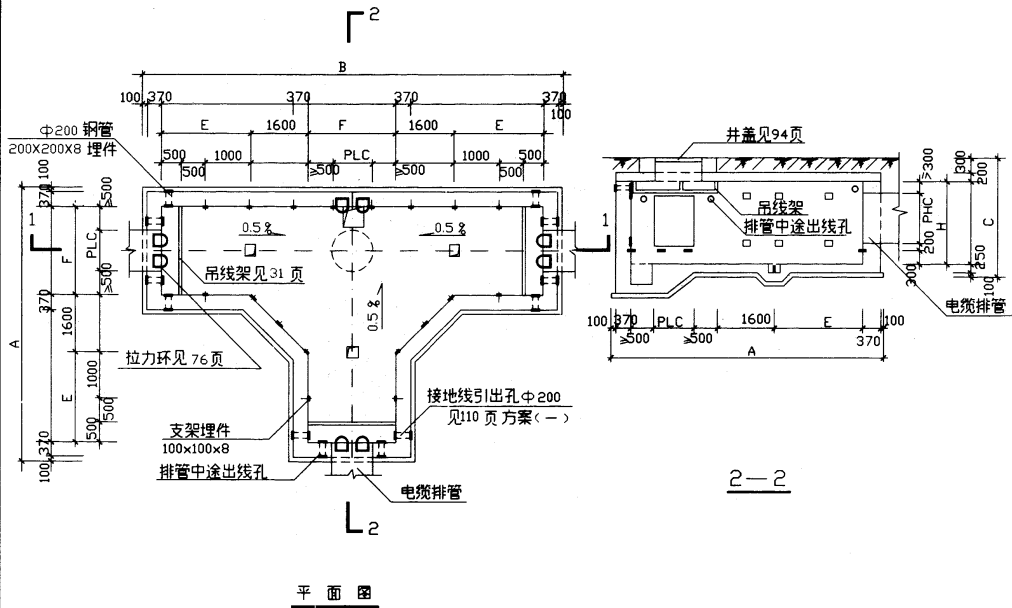
T形工作井平剖面(-)
