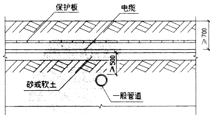
电缆与管道交叉(二)
