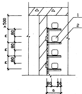
沿墙安装
