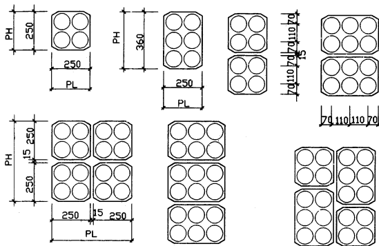
混凝土管块组合尺寸
