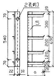
支架 5
