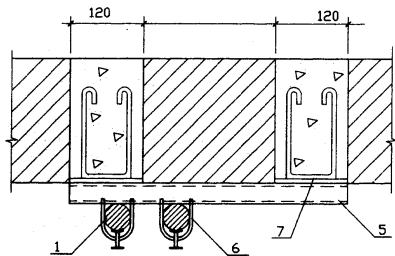
电缆在FJ-07、FJ-08型支架上敷设
