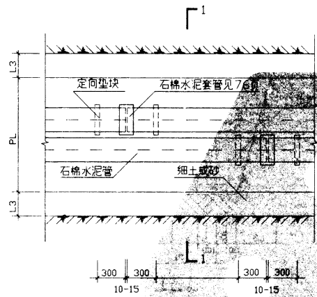
平面图
