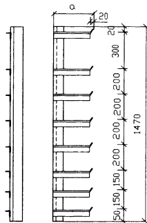
支架 4
