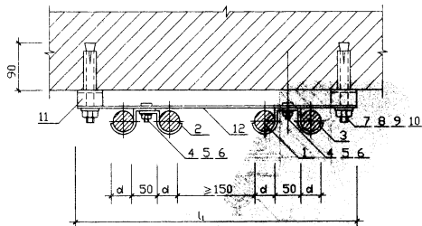
支架安装(一)
