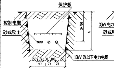
10kV 及以下电缆并列
