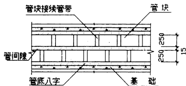
两行管块接缝错开
