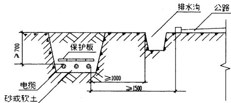
电缆与公路平行
