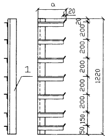
支架 1
