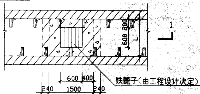
有覆盖层沟内集水井(双侧支架)
