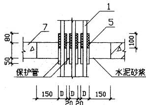
(四) 穿楼板保护管封堵
