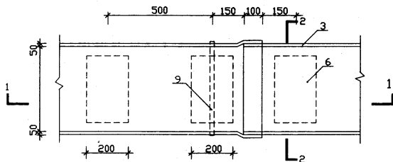
难燃封闭槽盒平面图
