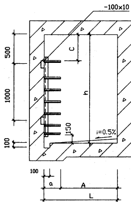
单侧支架
