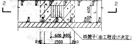
无覆盖层沟内集水井
