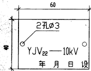
10kV及以上电力电缆标志牌
