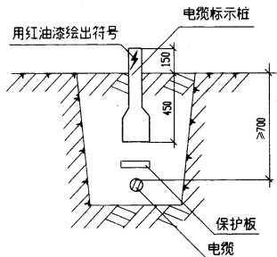
直埋电缆标示桩(-)
