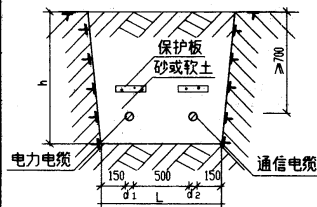
电力电缆与通信电缆并列(一)
