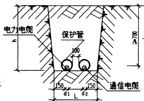
电力电缆与通信电缆并列(二)
