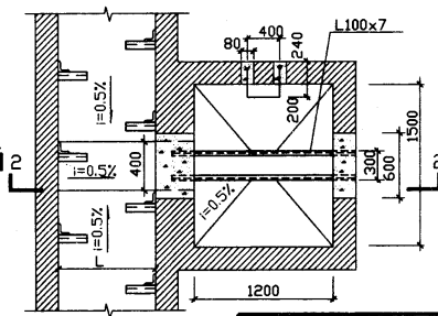
无覆盖层沟侧集水井
