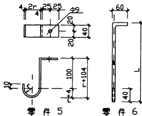
吊钩尺寸选择表
