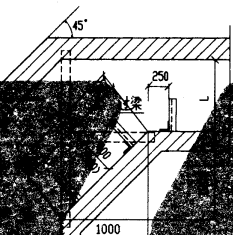
电缆沟转 45° (-)
