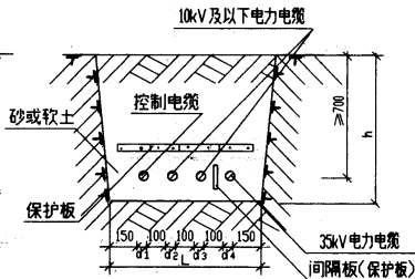
加间隔板电缆并列
