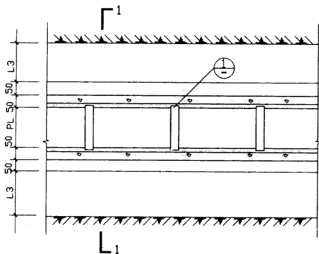
混凝土管块直埋平面
