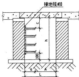
单侧支架电缆沟
