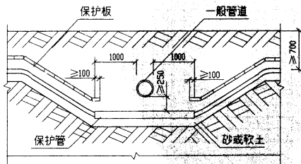
电缆穿管与管道交叉(一)
