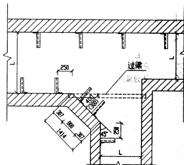
电缆沟分支段 (一)
