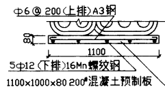
构件型式1 基础做法一
