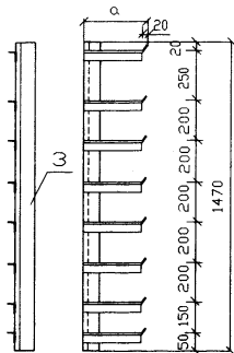
支架 3
