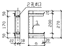
支架 1
