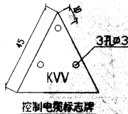
控制电缆标志牌
