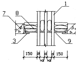
(三) 防火包封堵
