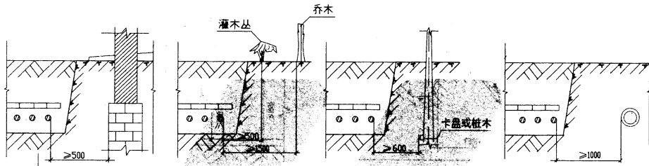
电缆与建筑物平行
