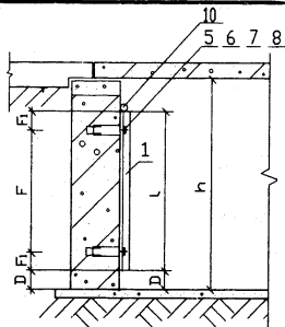
主架安装 (b)
