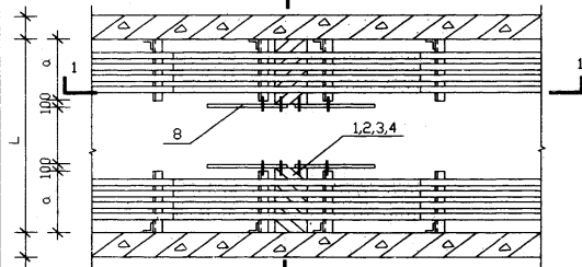
平面图
