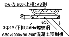
构件型式3 基础做法一
