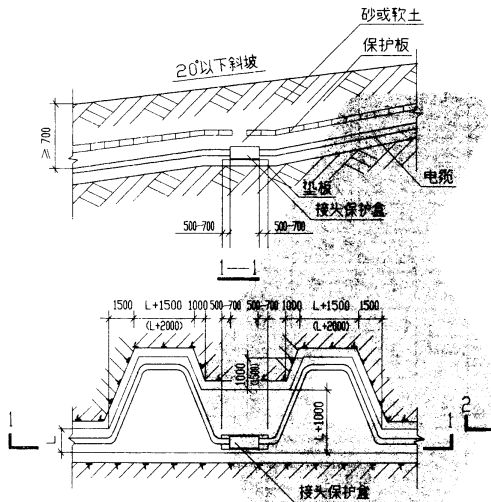
接头在 20^\circ 以下斜坡地段敷设
