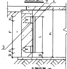
主架安装 (e)
