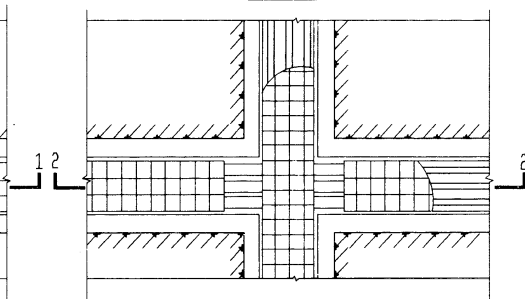
电缆与电缆交叉(二)
