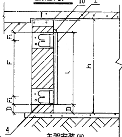
主架安装 (d)
