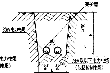
35kV 及以下电缆并列(二)
