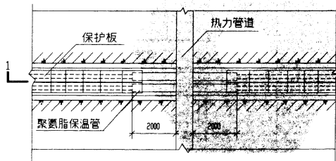
电缆与热力管道交叉(一)
