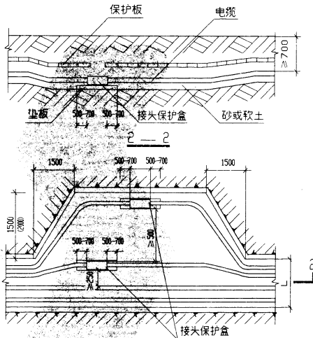
接头在水平地段敷设
