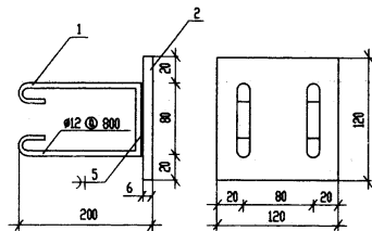
预埋件 1
