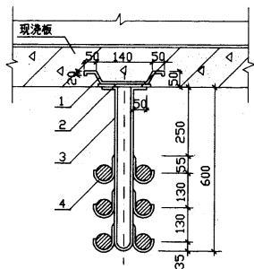
扁钢吊钩安装(一)
