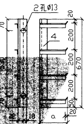
支架 4
