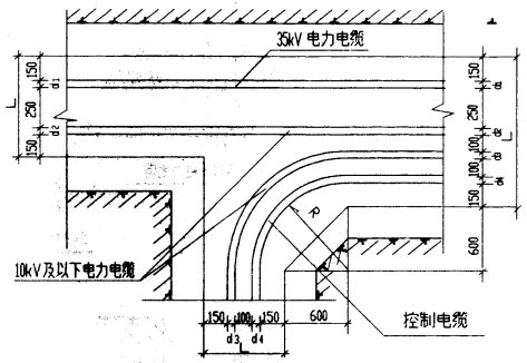
电缆直埋分支段(二)
