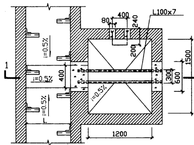
有覆盖层沟侧集水井
