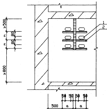
在电缆夹层中安装
