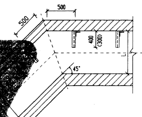
电缆沟转 45° (-)
