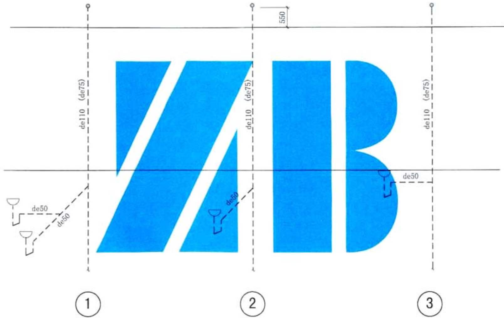
阳台雨落水系统图
