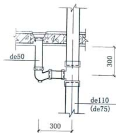
② 侧面
