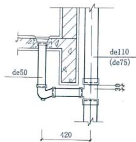
③ 立面
