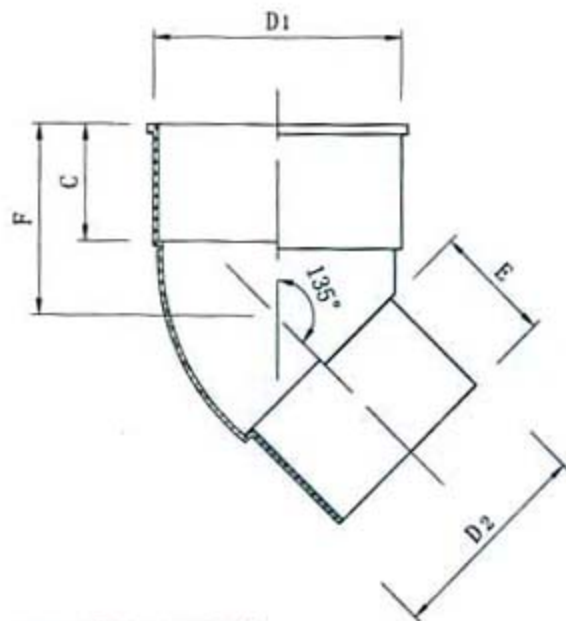
圆形管135°弯管
