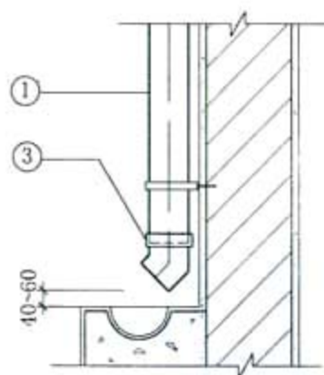
1 矩形管明沟排水
