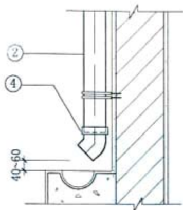
2 圆形管明沟排水
