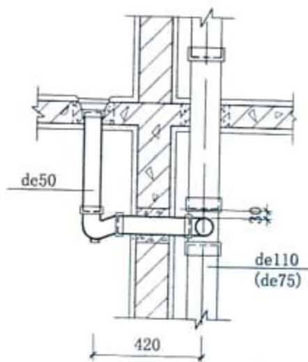
① 立面
