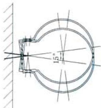
双支管卡安装
