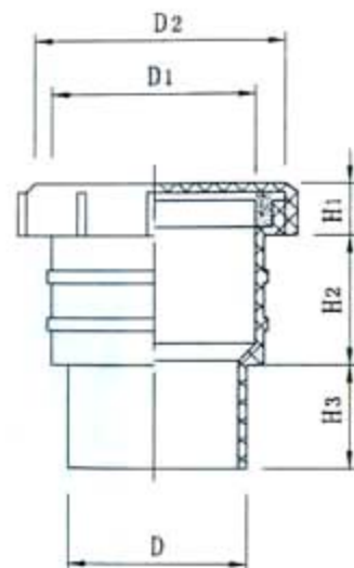
伸缩节
