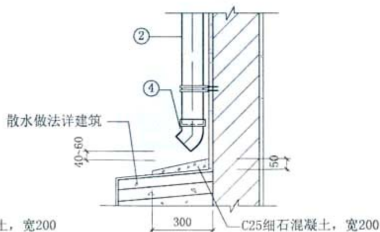
4 圆形管散水排水
