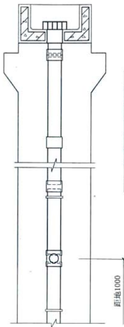
2 内排水安装图 (正立面)
